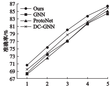
图6 5-way N-shot 下各模型准确率对比结果 (N 取值范围为 1 ~ 5)
