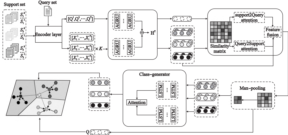
图 1 基于双向注意力和类生成器的小样本分类模型
