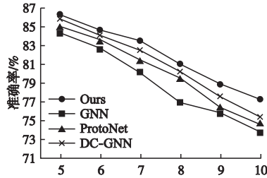
图5 N-way 5-shot 下各模型准确率对比结果 (N 取值范围为 5 ~ 10)
