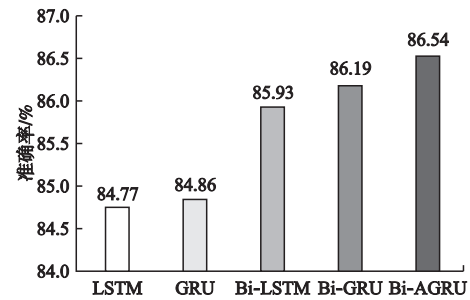
图 4 不同特征提取模块在 ARSC 数据集上的准确率
