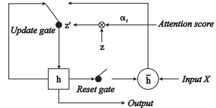
图 2 AGRU 结构图
